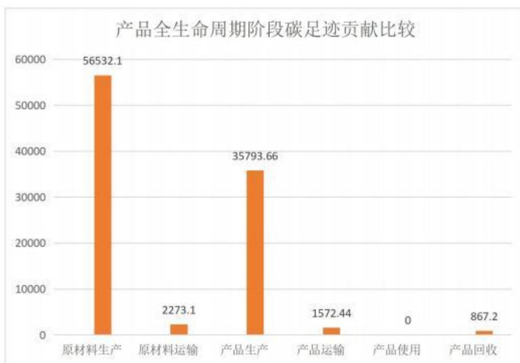
图 4 产品全生命周期阶段碳足迹贡献图
