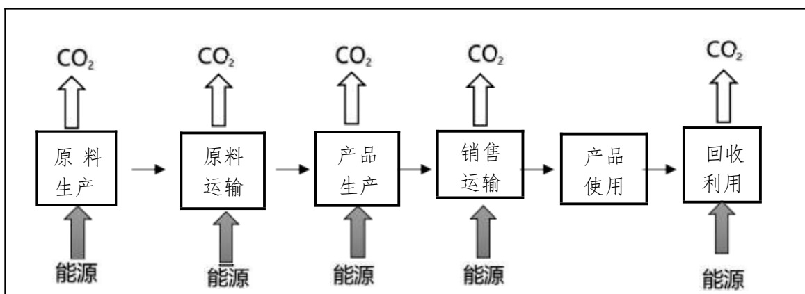
图 2 原料药产品生命周期评价边界图
