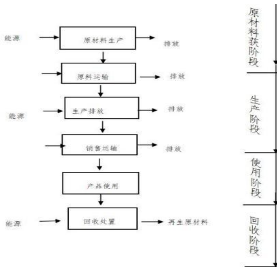
图 1 原料药生命周期系统边界图
